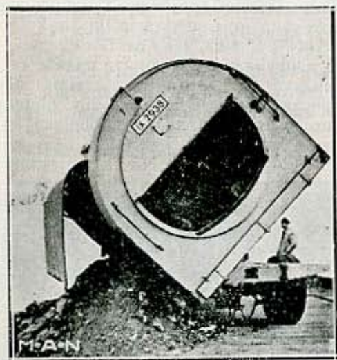
Сл. 18. — Аутомобил за смешлиште фирме М.А.Н.
