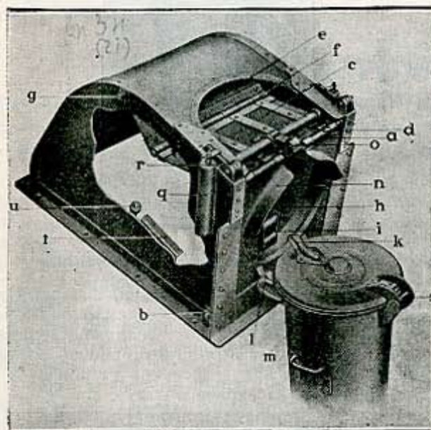
Сл. 21. — Затварач „Es—Em“ у тренутку кад се суд закљони
