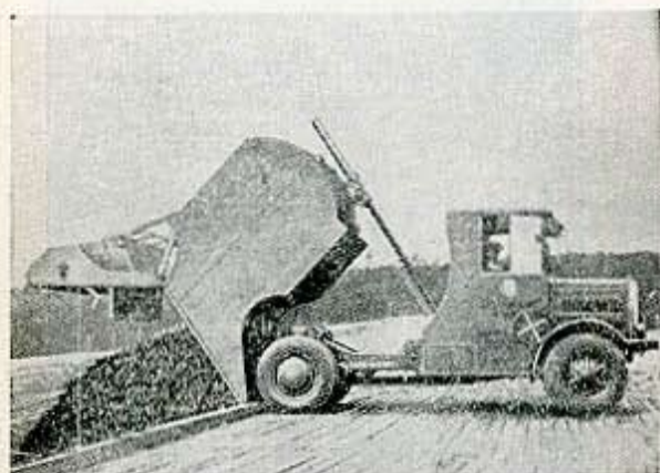
Сл. 17 а. — Изручивање смешлишта аутомоб. Faun
