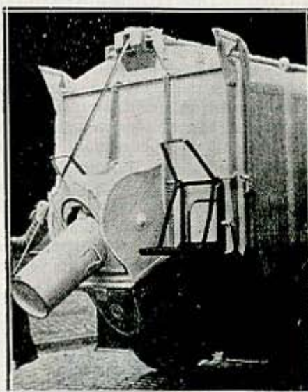
Сл. 20. — Аутомобил са затварачима
