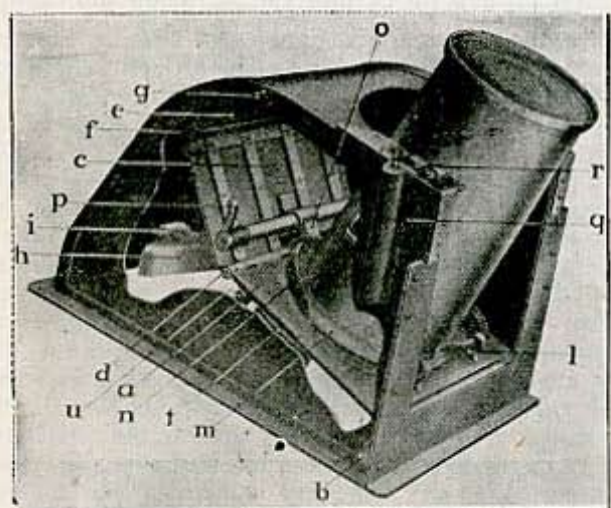
Сл. 22. — Затварач „Es—Em“ у тренутку кад се суд изручује
