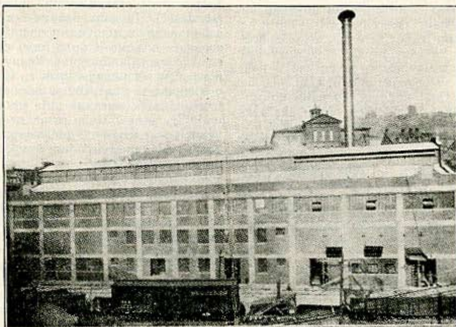
Забод за сагоревање и утилизацију ђубришта у Питсбургу, који по типу и димензијама одговара Забоду потребном за Београд
