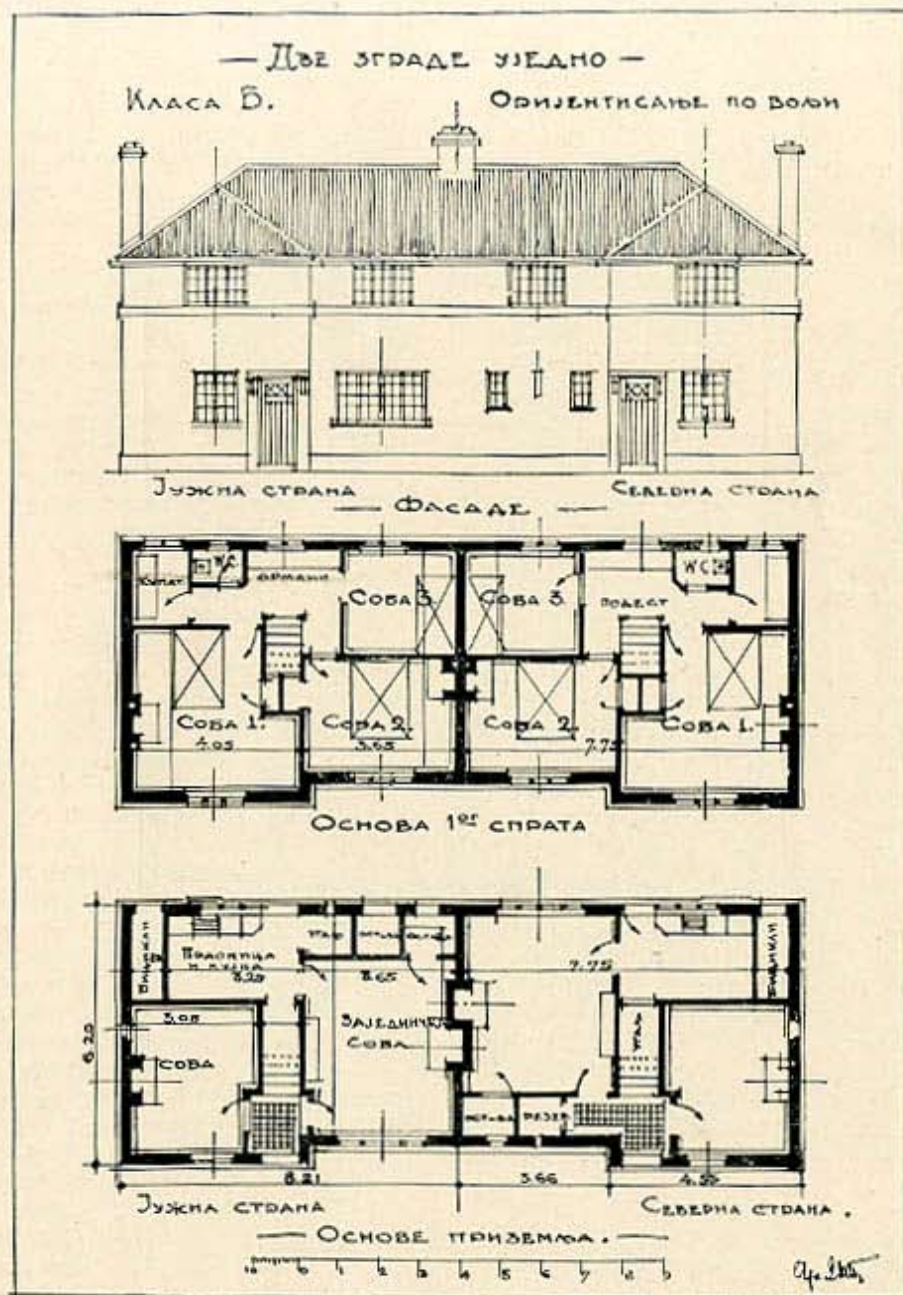
Тип зграде коју је предложило енглеско Мин. Нар. Здравље. Тип Б
