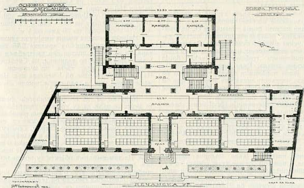
Основна школа „Краља Александра I.“ — Основа приземља
