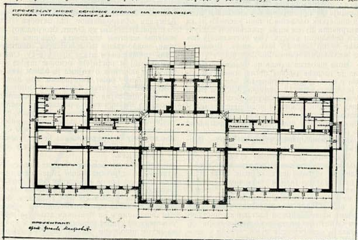
Основна школа на Вождовцу. — Основа приземља
