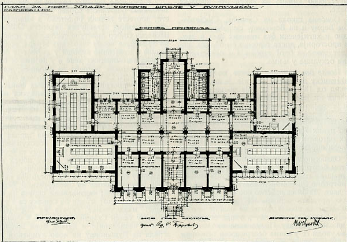
Основна школа у Булбулдеру. — Основа приземља
