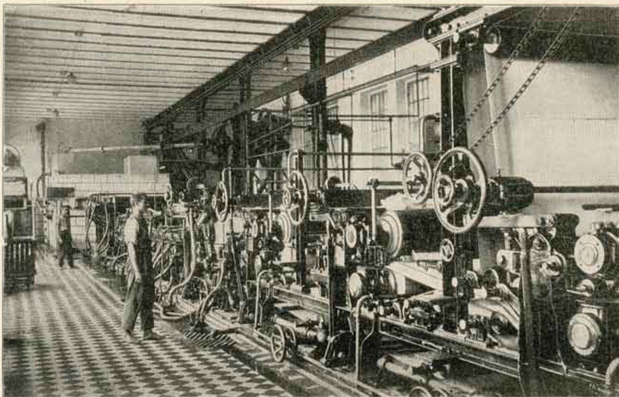
I део машине за израду хартије
