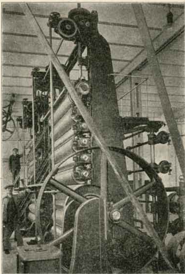
Каландер за сатинирање хартије
