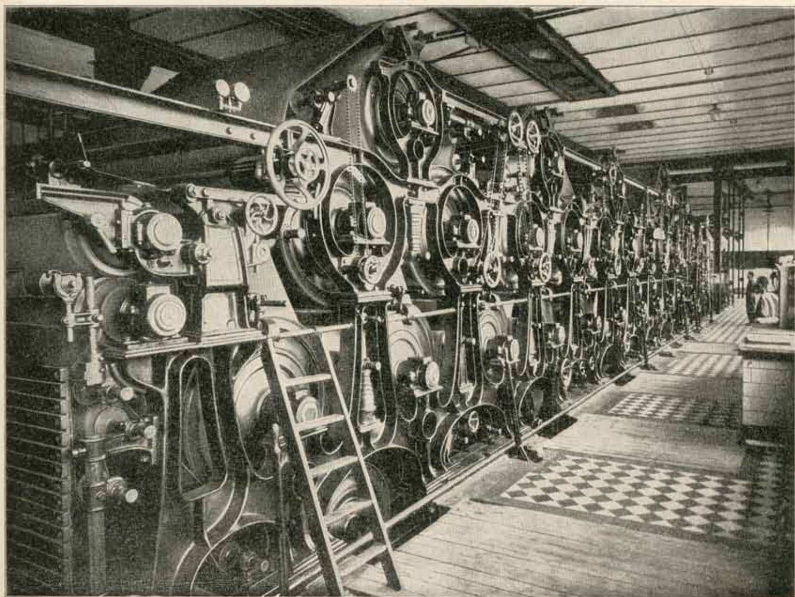
II део машине за израду хартије
