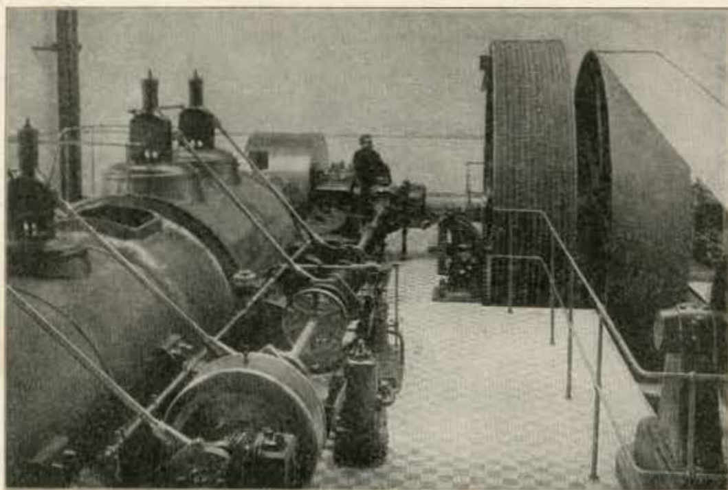
Фабричка електрична централа од 1000 коњских снага са генератором од 500 коњских снага
