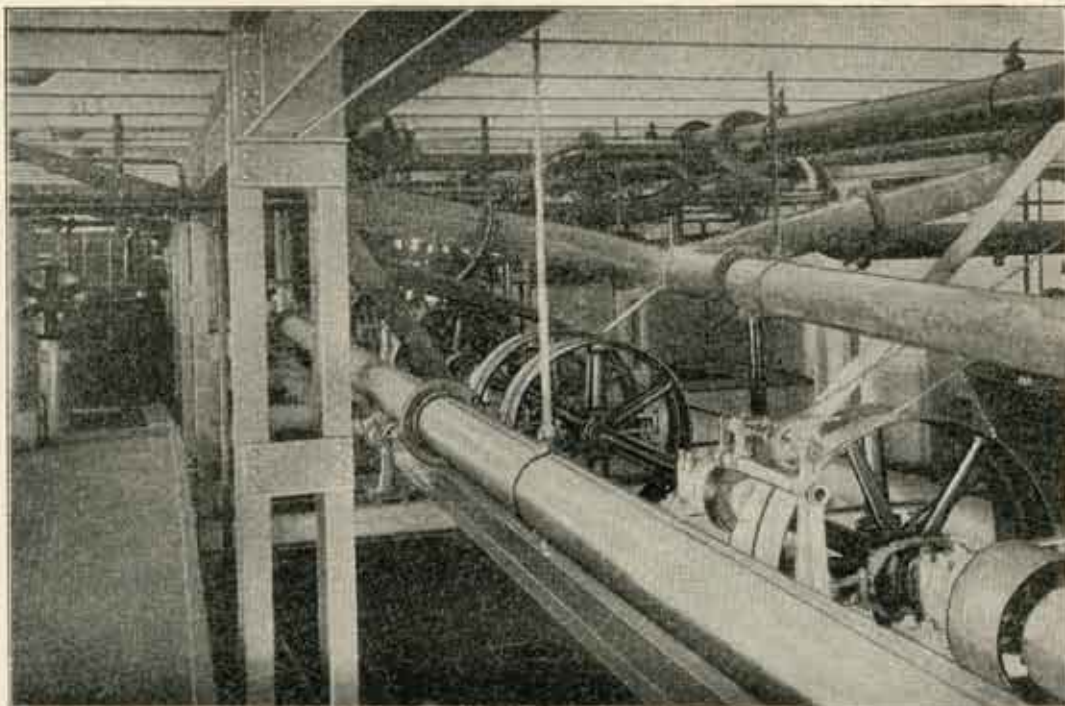
Главна трансмисија
