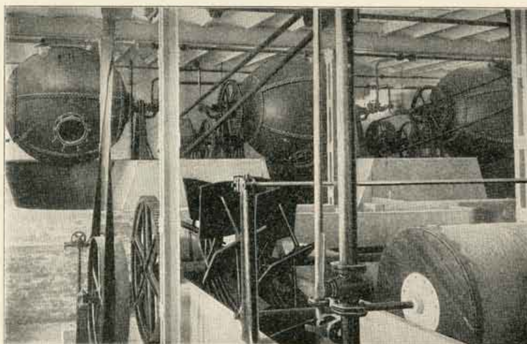
Казани за кување крпа и осталог материјала
