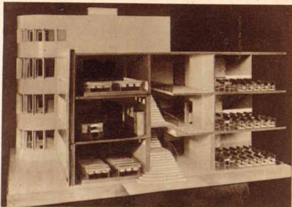
Пројекат за школу у Дителну по нацрту арх. Вала и Редела. Зграда: армиран бетон, намештај, врата и провори од челика
